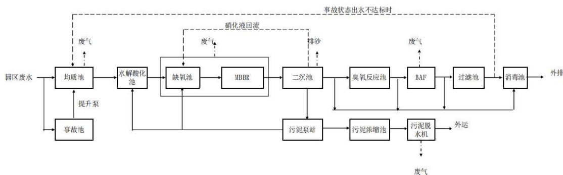
图 6.1-1 污水处理厂处理工艺流程图
