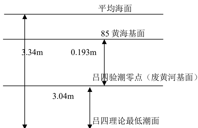
图 4.1-15 基准面关系图
