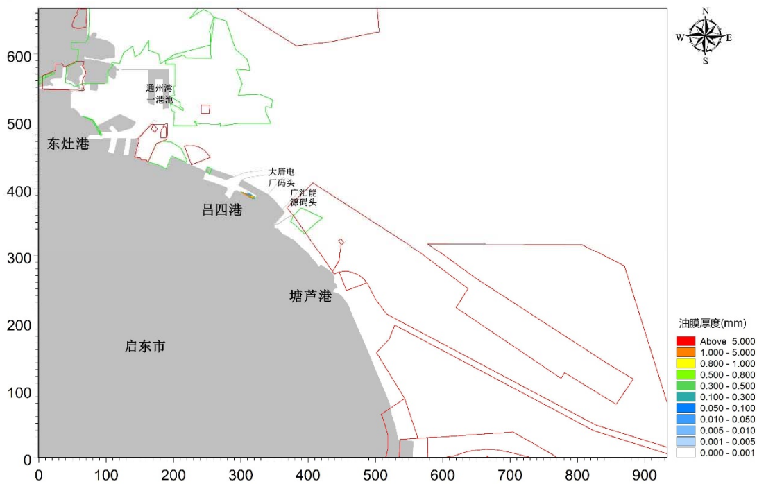
图 5.10-3 工况 2 条件下码头附近船舶溢油后 72 小时内油膜的扫海范围 (红线区：海洋生态红线；绿线区：养殖区)
