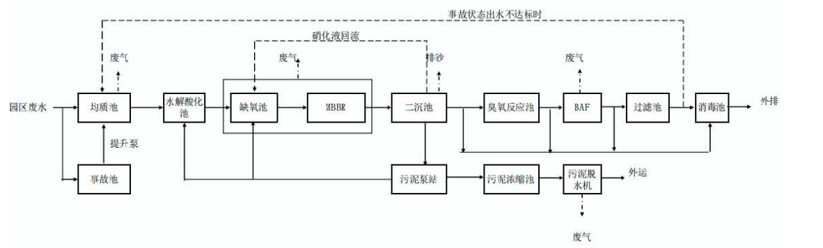
图 6.1-3 污水处理厂处理工艺流程图
