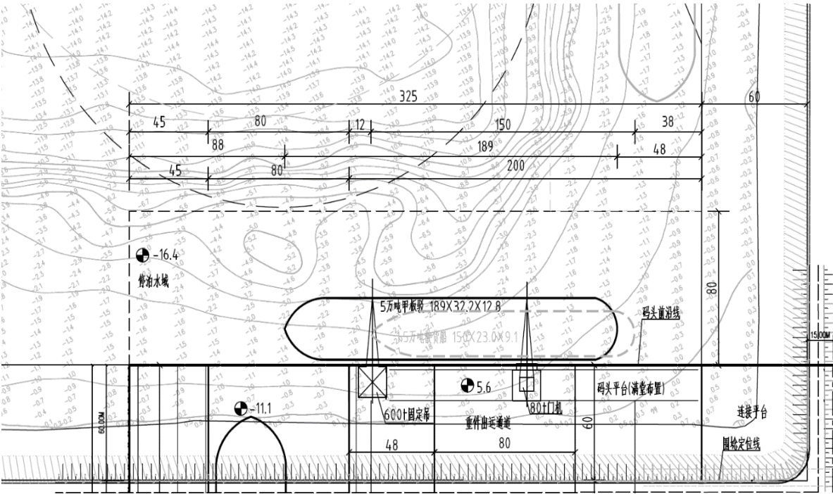
图 3.1-10 码头前沿现状地形分布图
