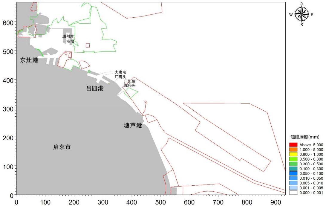
图 5.10-4 工况 3 条件下码头附近船舶溢油后 72 小时内油膜的扫海范围 (红线区：海洋生态红线；绿线区：养殖区)
