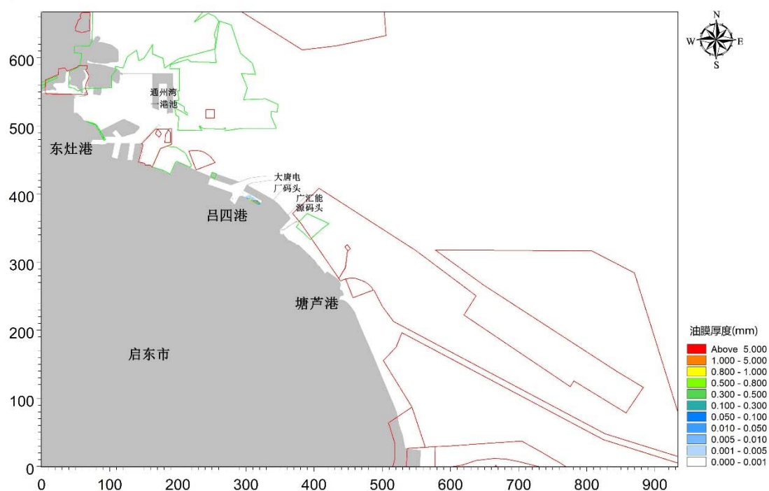
图 5.10-2 工况 1 条件下码头附近船舶溢油后 72 小时内油膜的扫海范围 (红线区：海洋生态红线；绿线区：养殖区)
