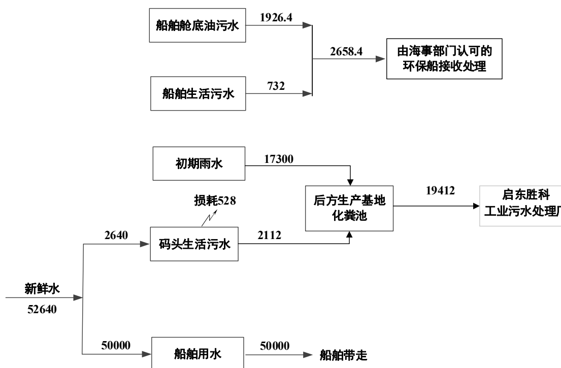
图 3.3-1 运营期水平衡图 (t/a)
