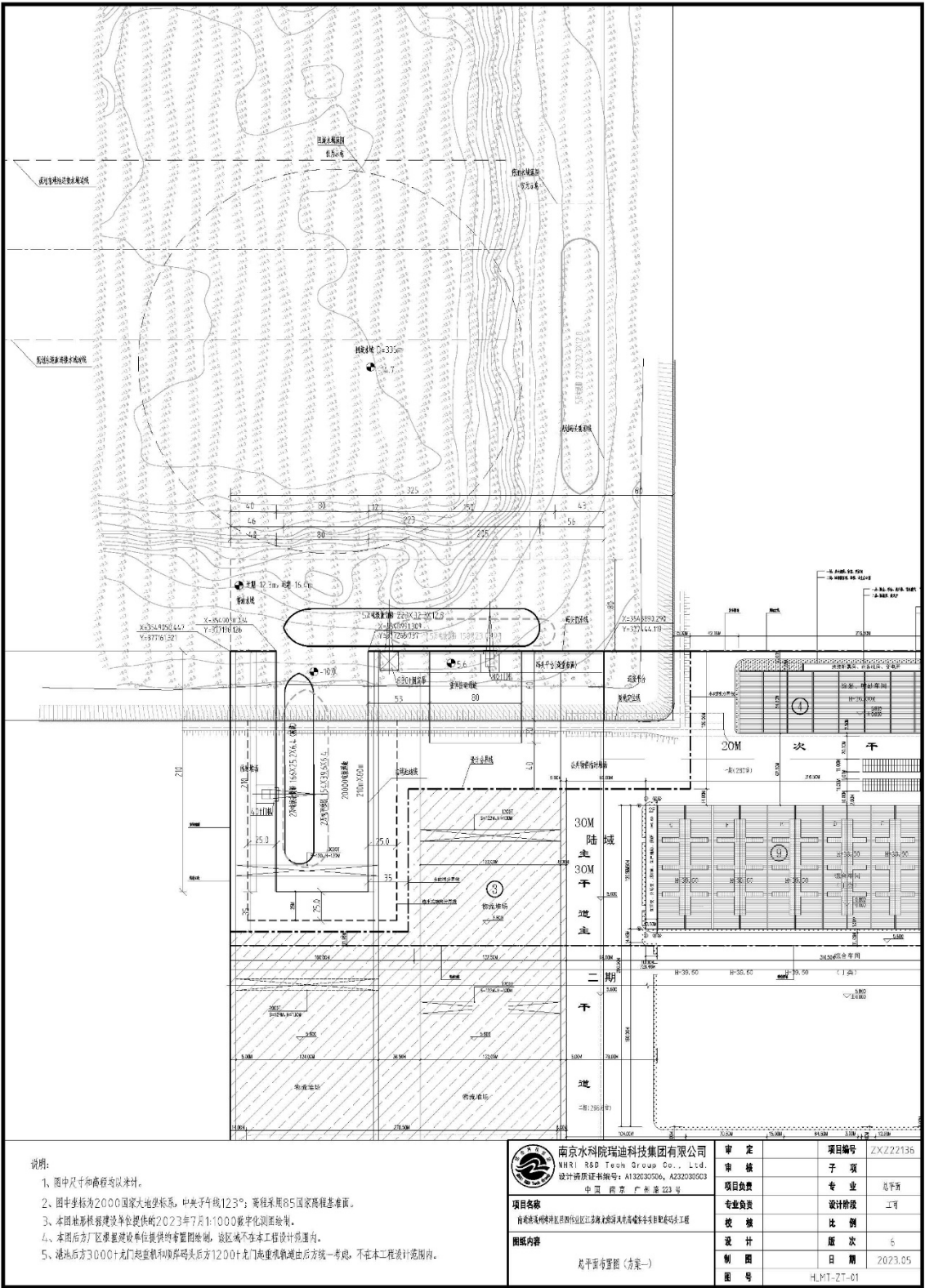
图 3.1-17 本项目总平面布置图 (含地形图)
