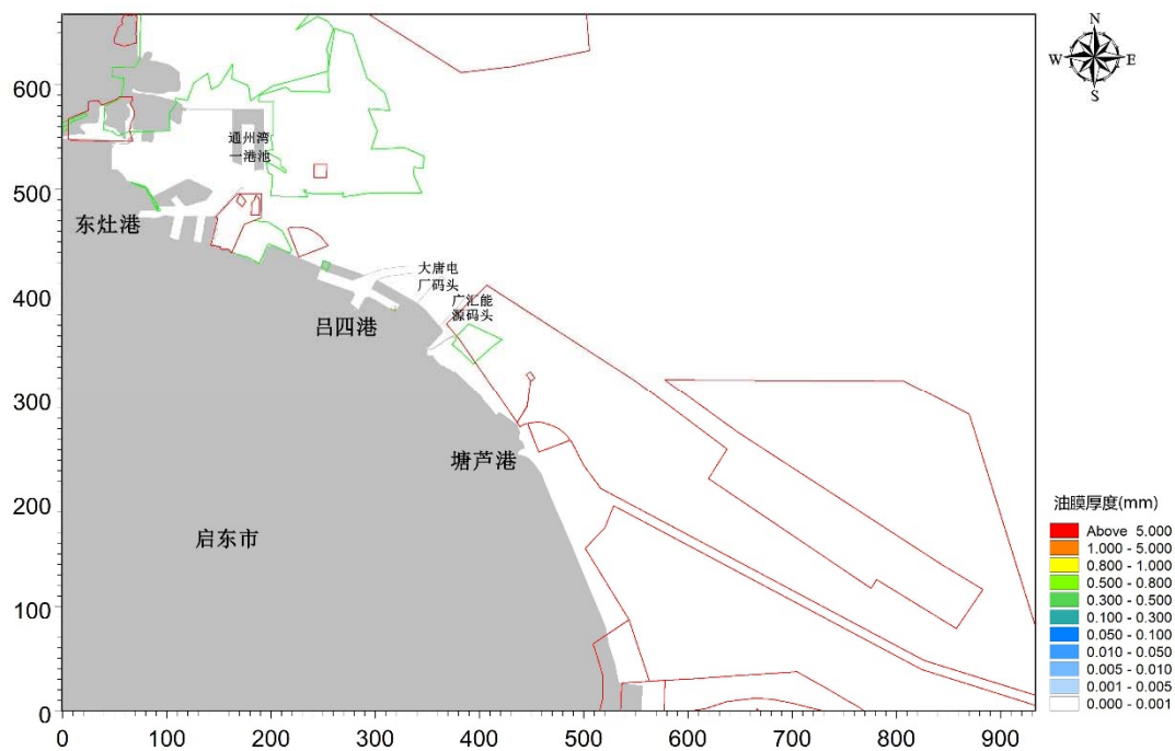
图 5.10-5 工况 4 条件下码头附近船舶溢油后 72 小时内油膜的扫海范围 (红线区：海洋生态红线；绿线区：养殖区)
