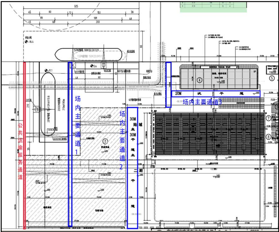
图 3.1-9 码头装卸运输通道示意图
