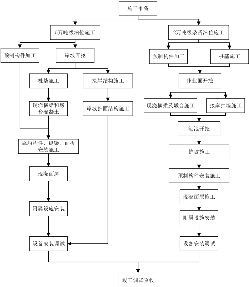
图 3.2-2 码头总体施工流程图
