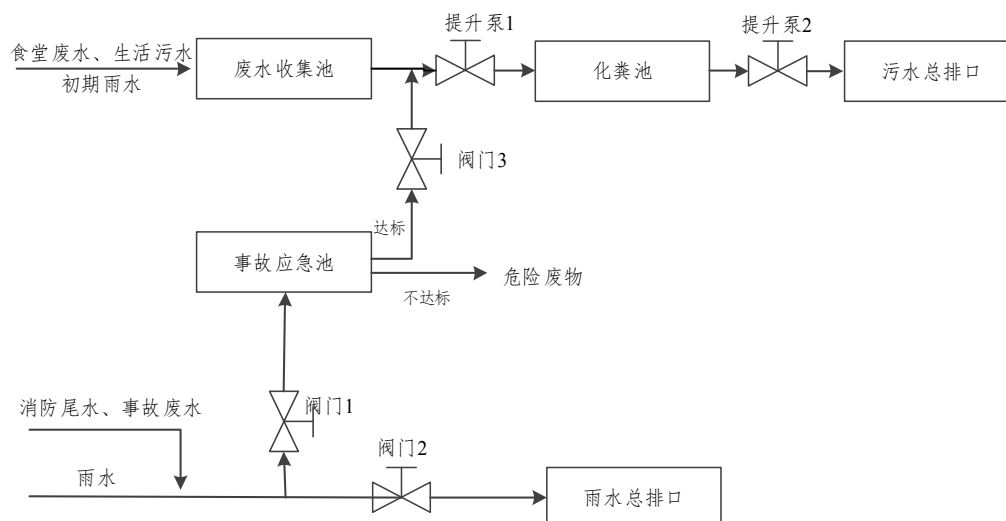
图 6.3-1 事故情况各废水截留走向图
