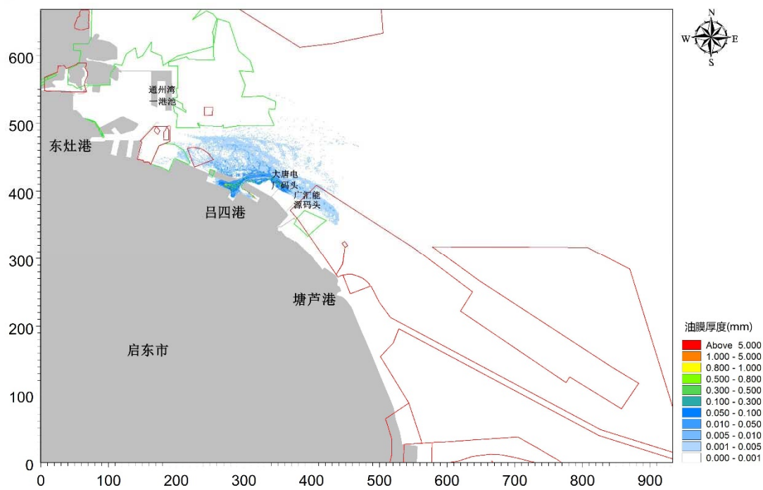
图 5.10-6 工况 5 条件下码头附近船舶溢油后 72 小时内油膜的扫海范围 (红线区：海洋生态红线；绿线区：养殖区)
