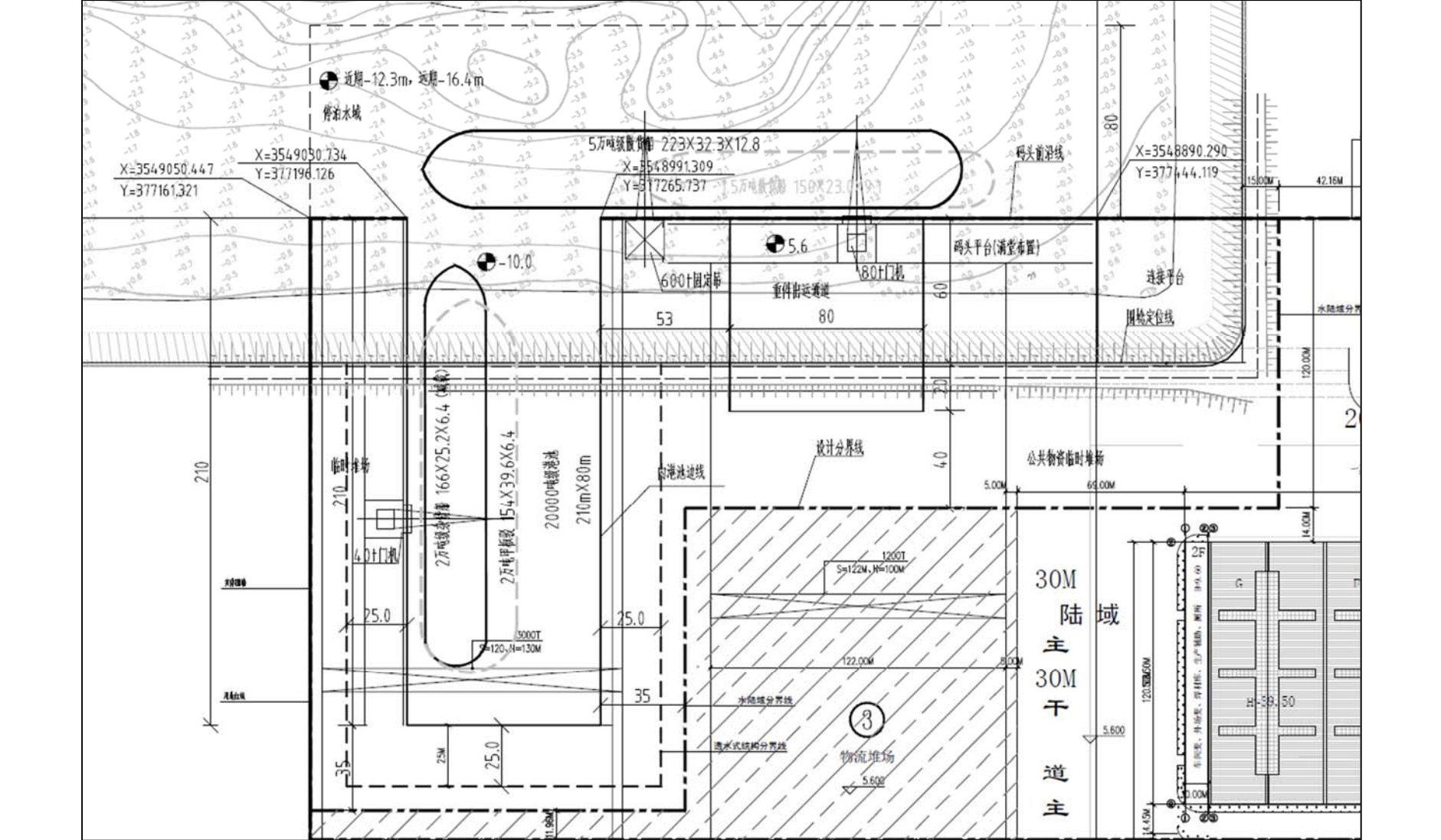
图 3.1-16 码头平面布置图 (含地形图)
