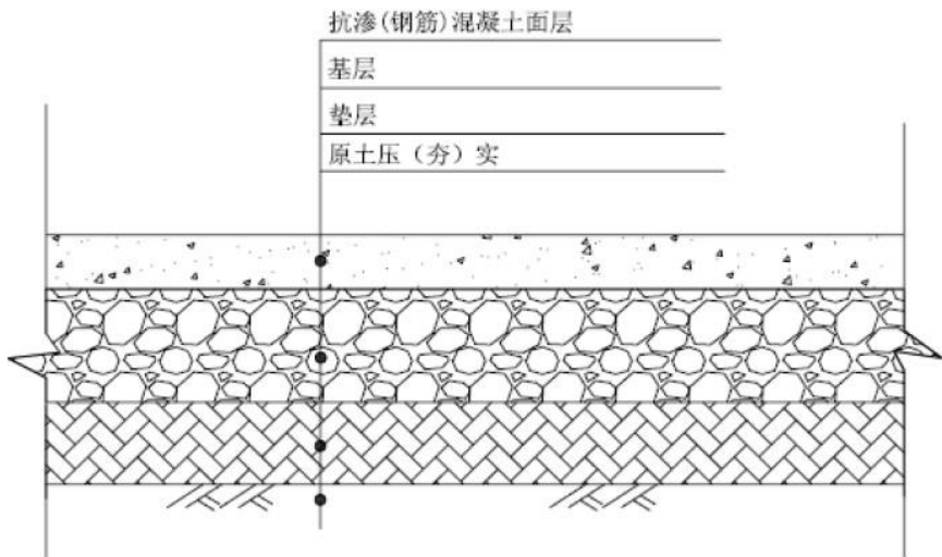
图 7.5.2-1 一般防渗区域防渗结构
