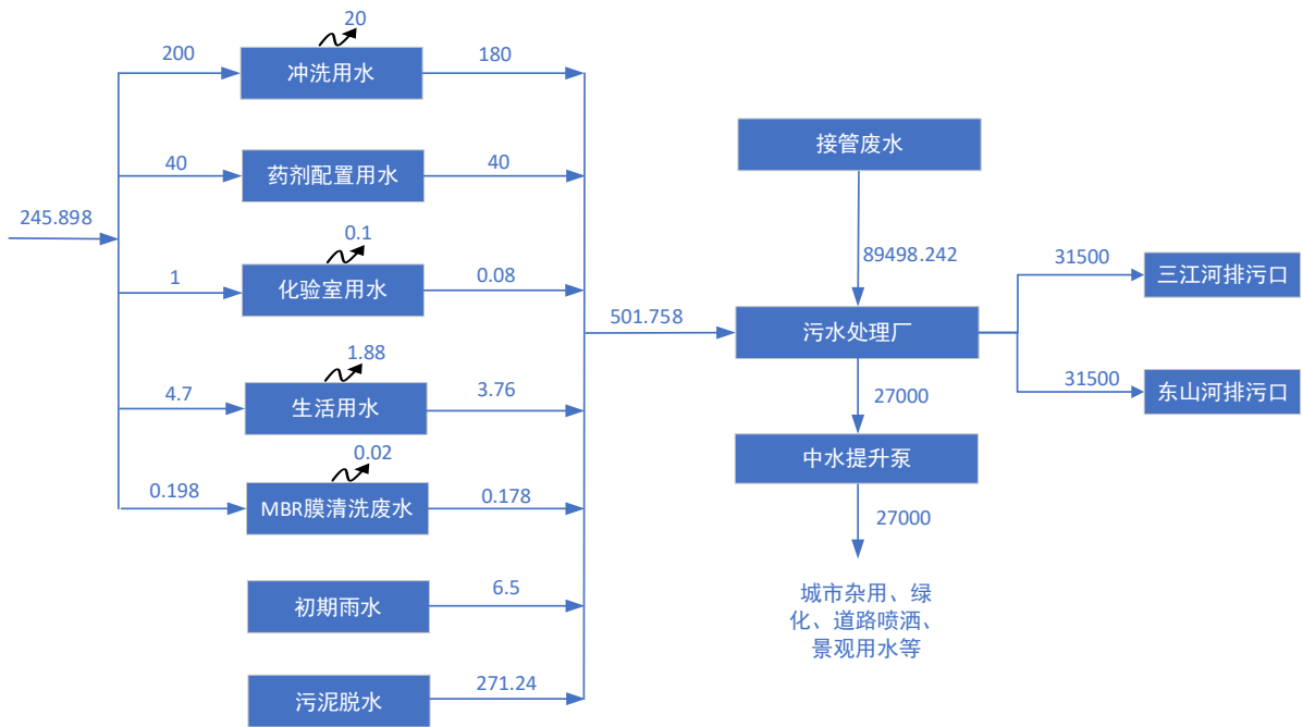
图 4.3-2 本项目建成后全厂水平衡图 ( \text{m}^3/\text{d} )
