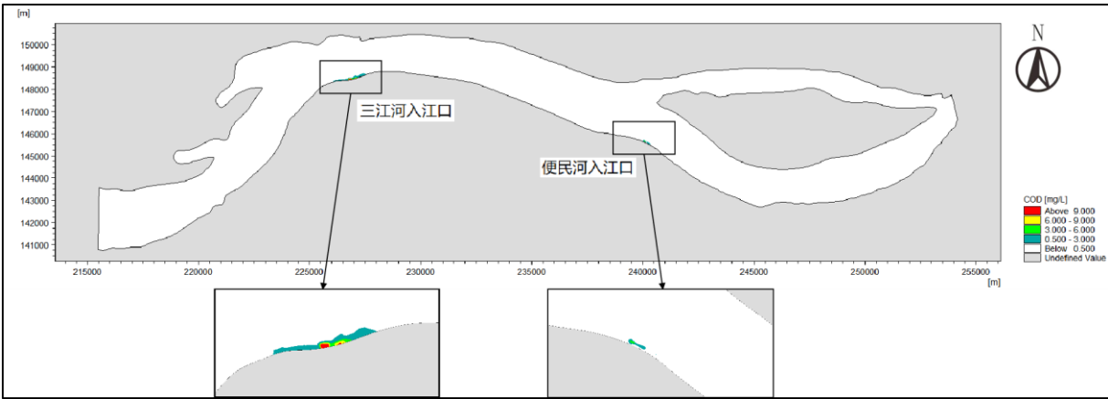
图 6.2.8-2 工况 2COD 最大浓度包络线图
