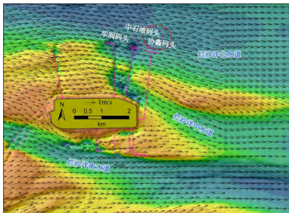
图 3-7.2 工程局部流态图（落急时刻）
