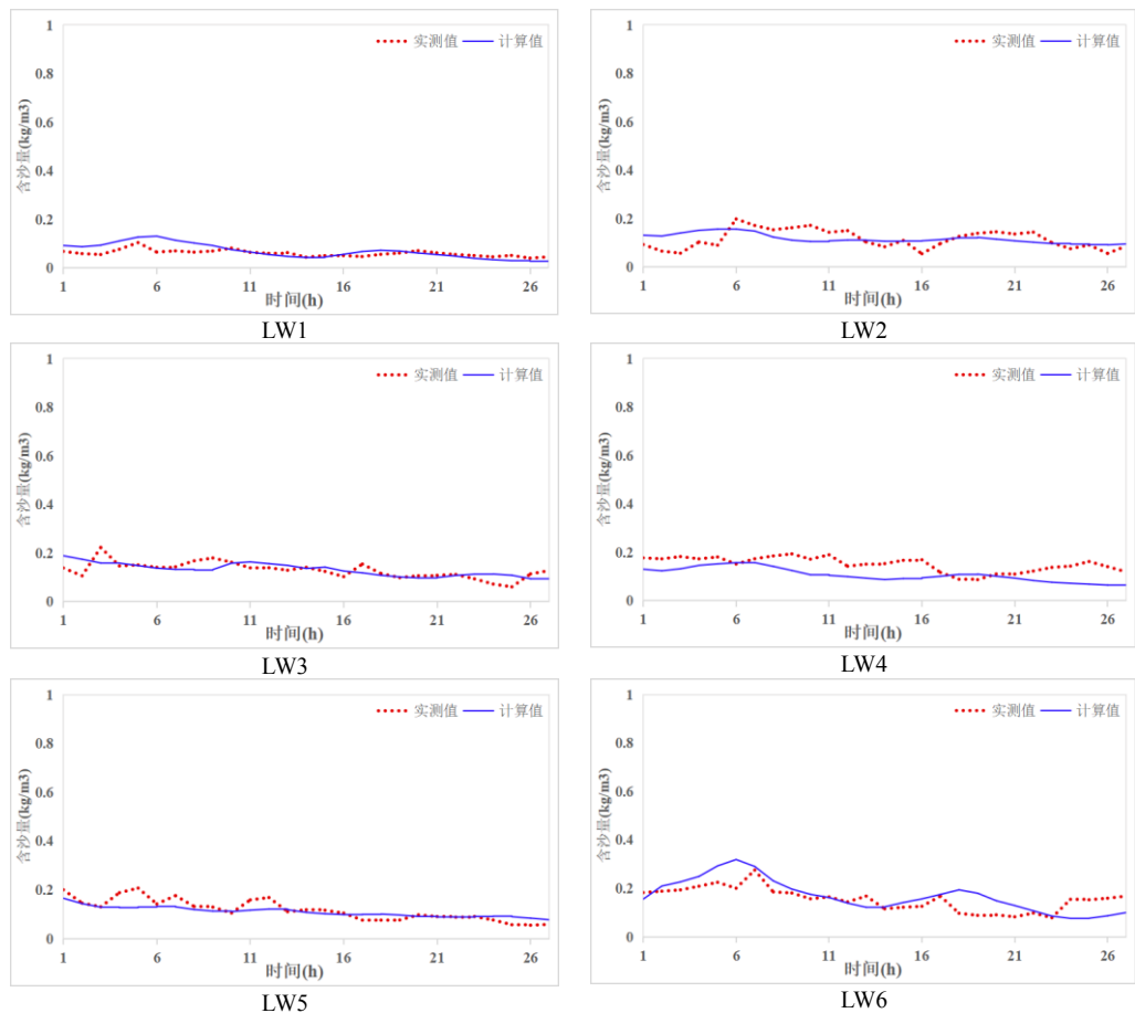
图 5.1-8 小潮含沙量过程验证
