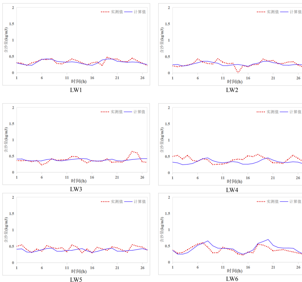
图 5.1-7 大潮含沙量过程验证
