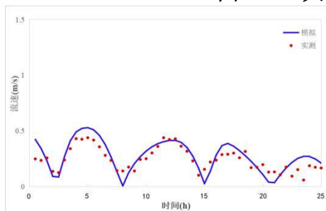
图 5.1-5 大潮流速流向验证
