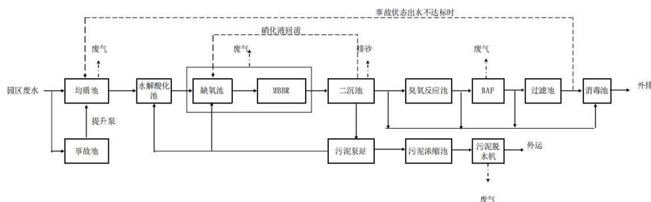
图 6.1-1 污水处理厂处理工艺流程图
