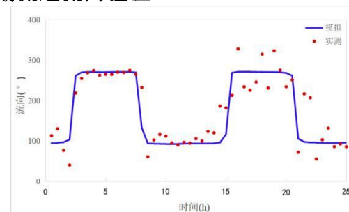
图 5.1-5 大潮流速流向验证
