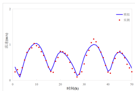
图 5.1-5 大潮流速流向验证
