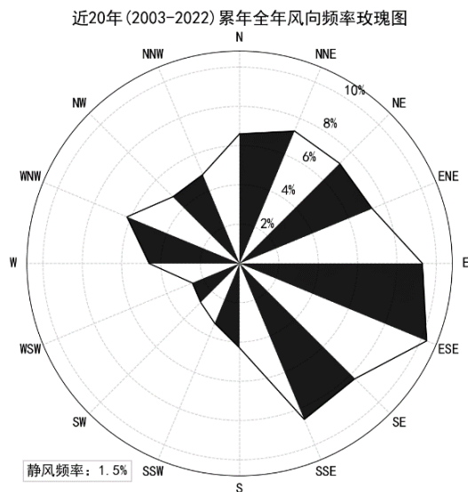
图 4.1-2 吕四气象站风玫瑰图
