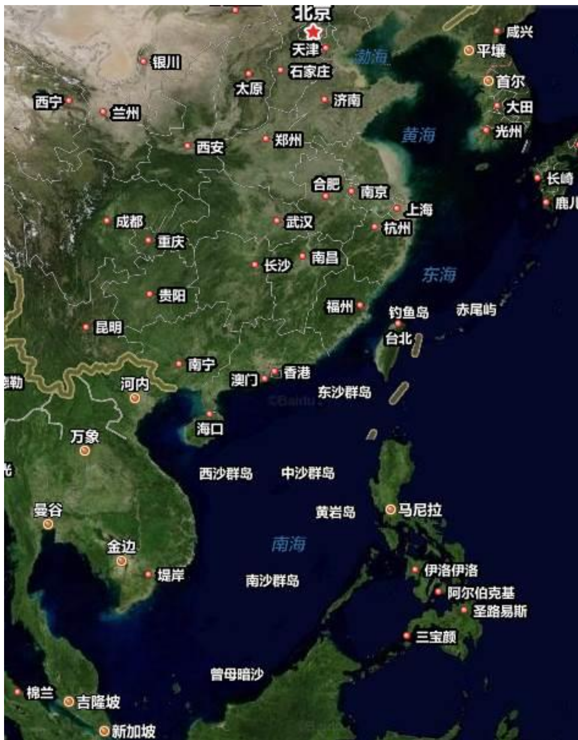
图 5.1-1 中国近海潮波模型研究海域示意图
