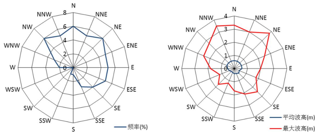
图 4.1-19 吕四海洋站波浪玫瑰图（1969 年～2001 年）
