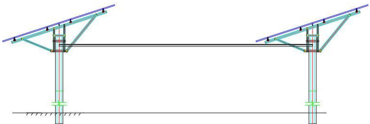
图 2-4 桥架安装示意图
