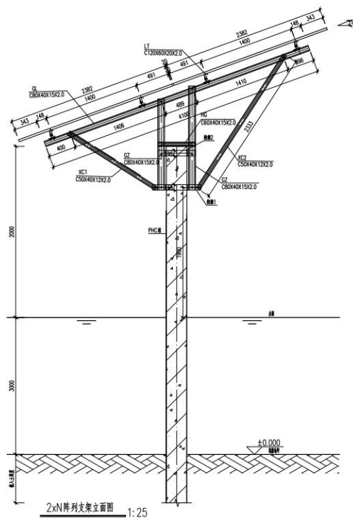
图 2-3 2×N 阵列支架立面图
