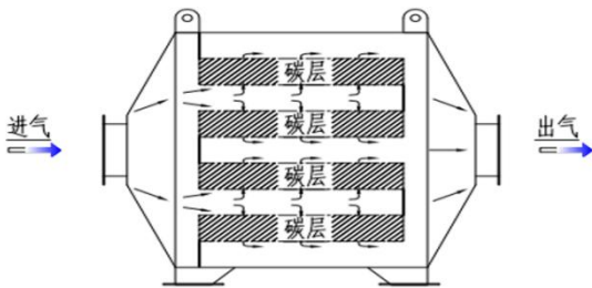
图 4-3 活性炭吸附装置效果图
