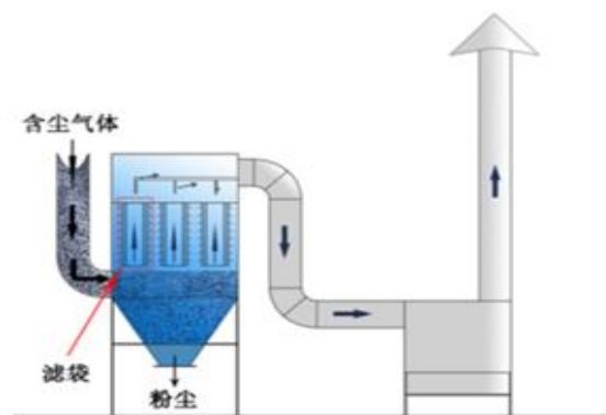
图 4-2 布袋除尘器效果图
